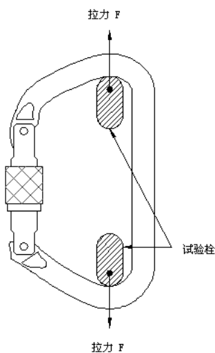
图1 安全钩开口闭合状态长轴方向破断强度测试示例
